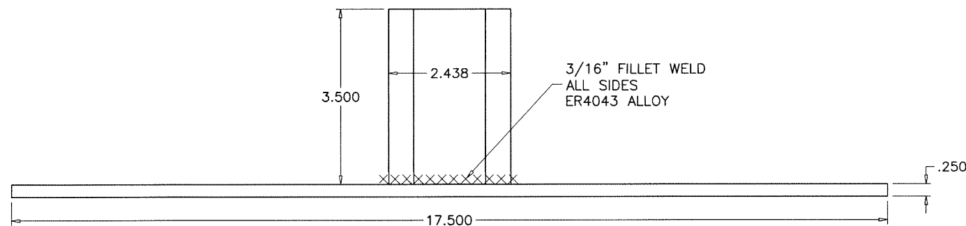
10A 'T' ANCHOR
