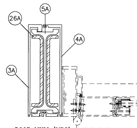
DOOR MULL 'MD5'
